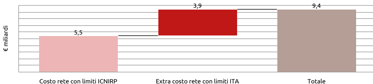
Figura 5.11 Costo di upgrade della rete al 5G in relazione ai limiti elettromagnetici (2018)
